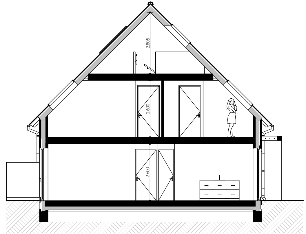
Doorsnede
