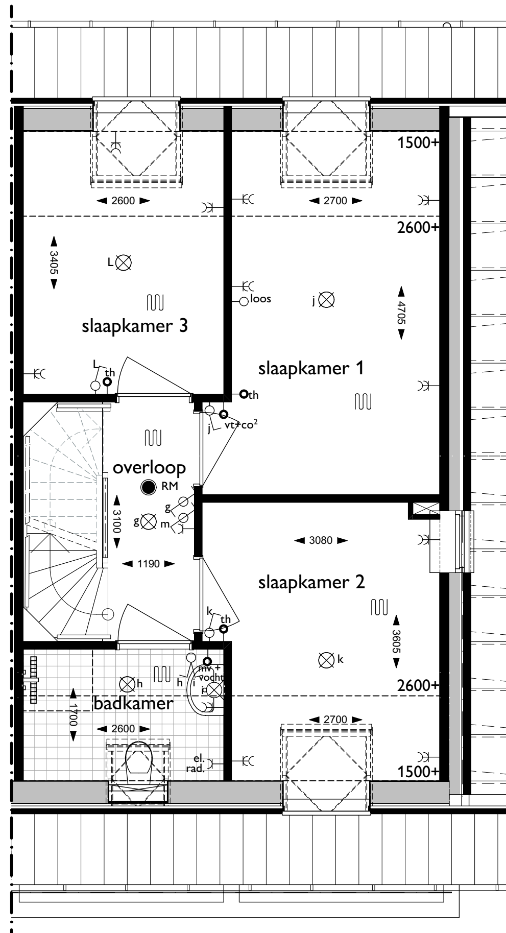
Eerste verdieping
