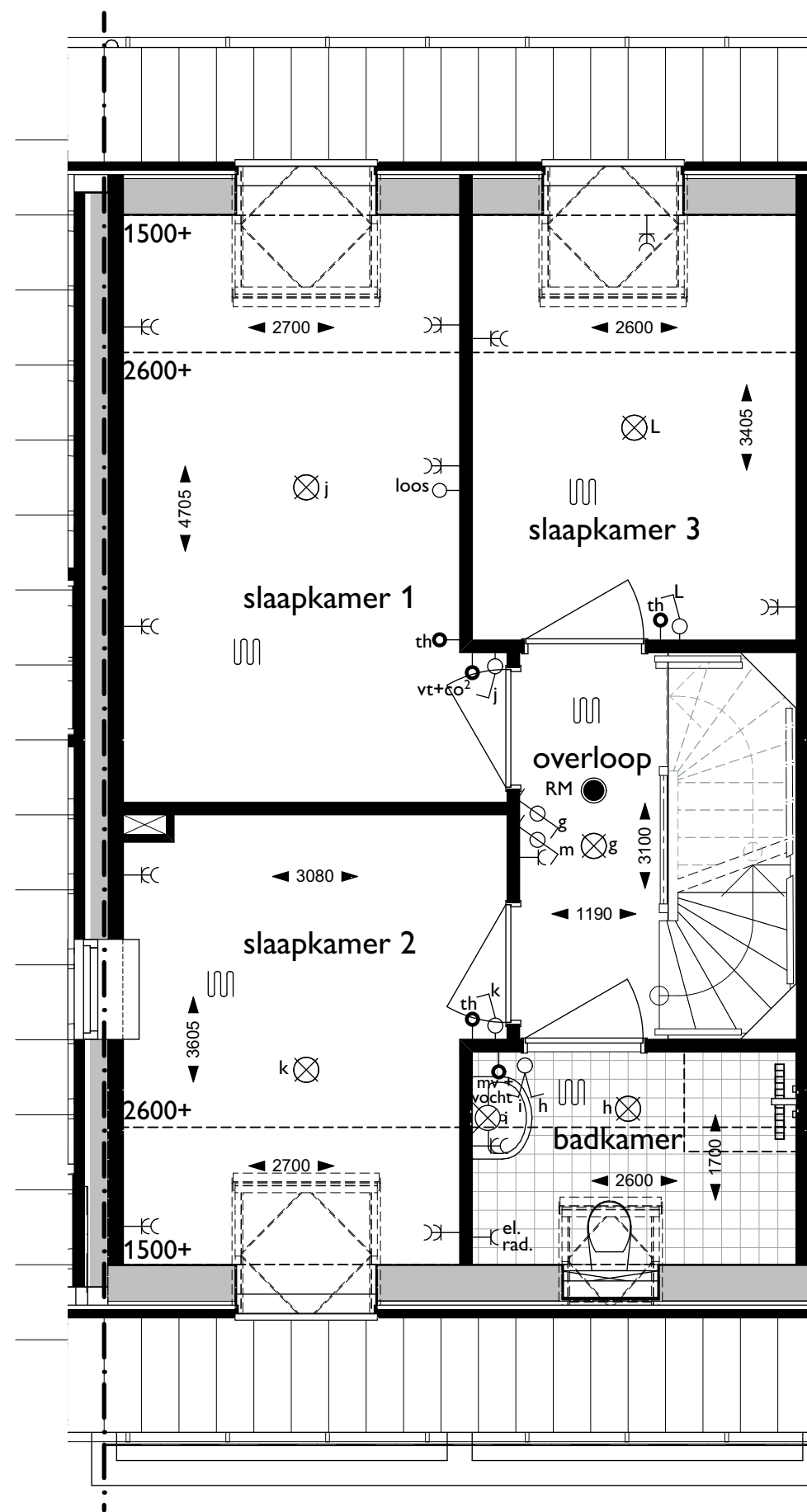
Eerste verdieping
