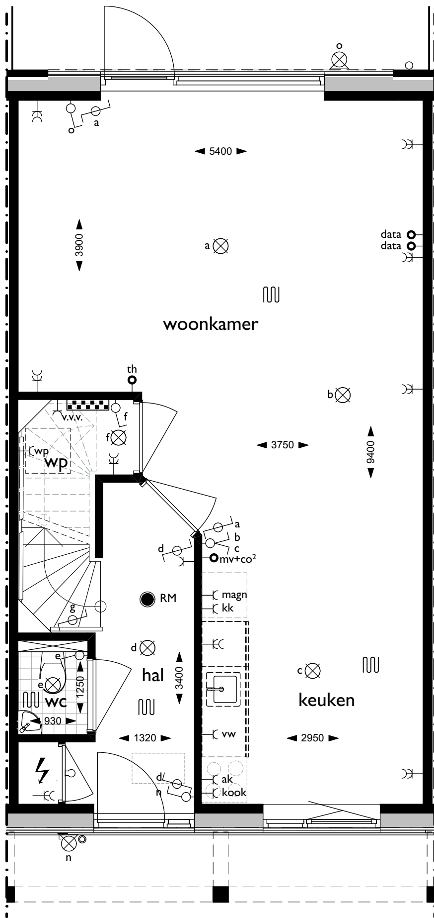
Begane grond
