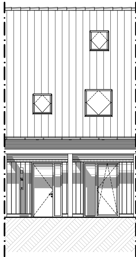
Vorgevel
