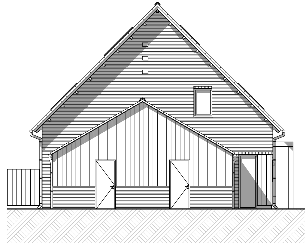
Linkergevel
