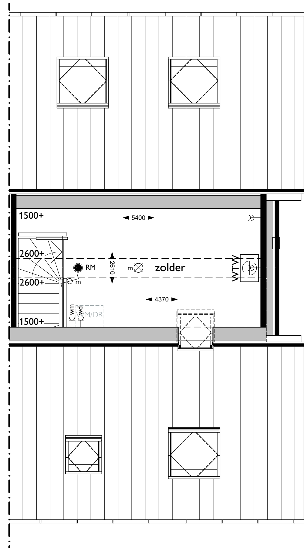
Tweede verdieping
