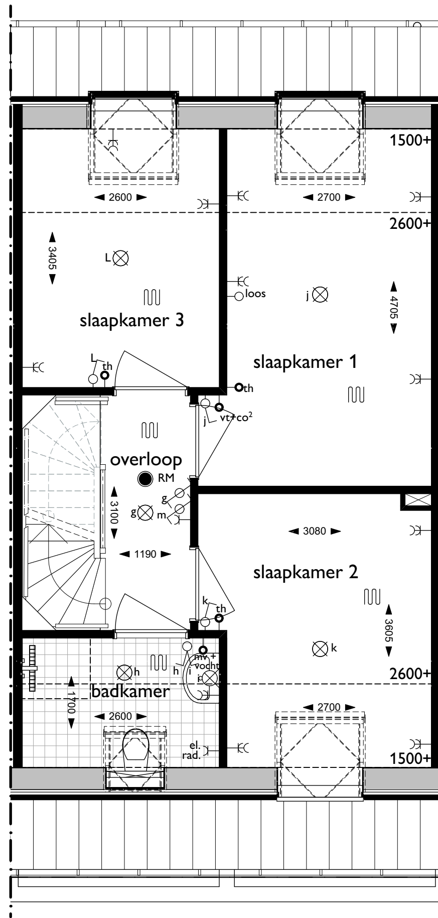
Eerste verdieping
