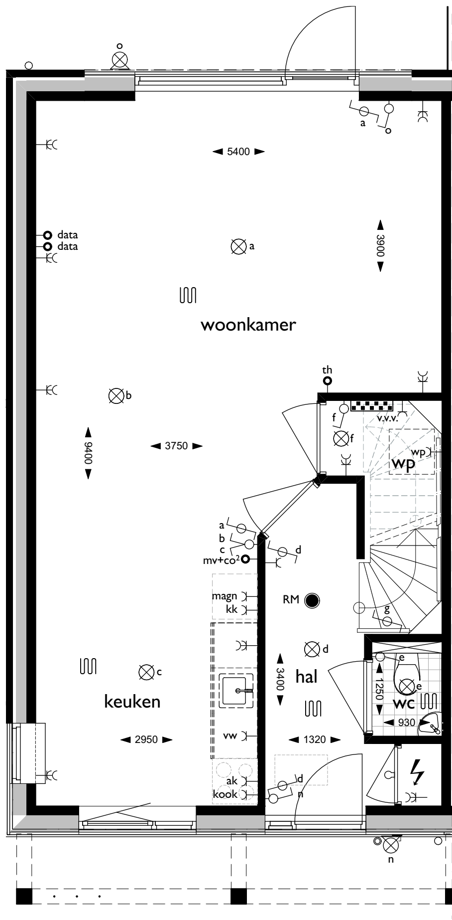
Begane grond
