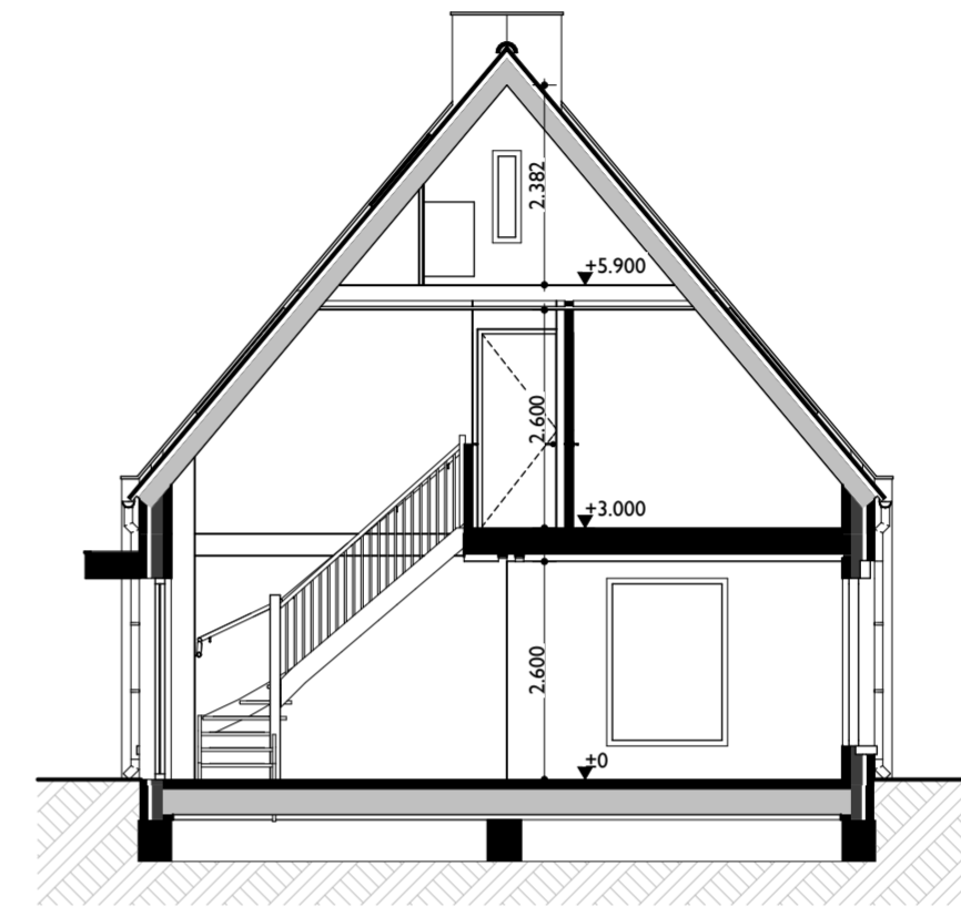
Dwarsdoorsnede
