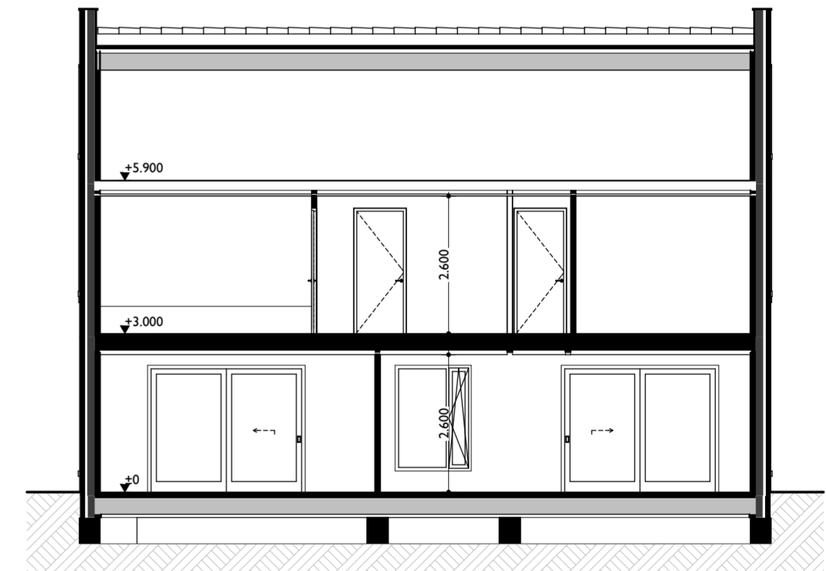
Langdoorsnede
