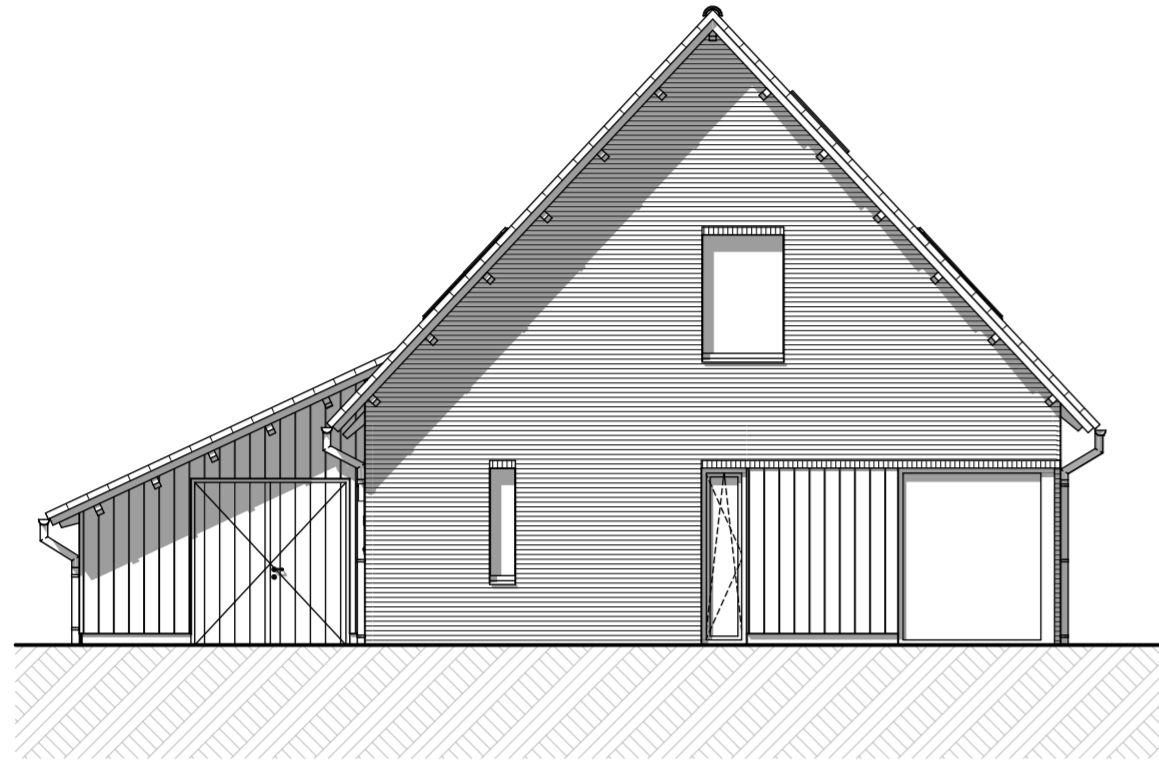
bnr 1/2 Vorgevel
