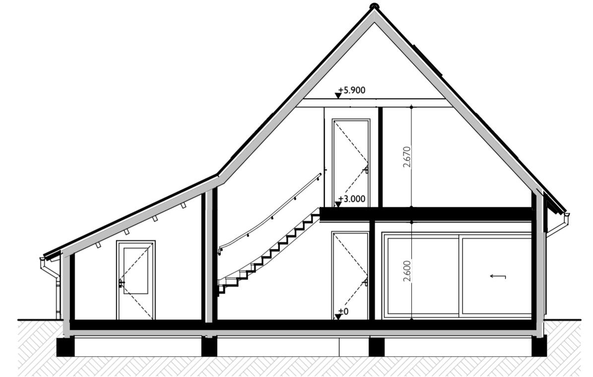
Dwarsdoorsnede
