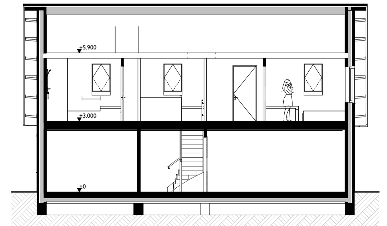
Langsdoorsnede
