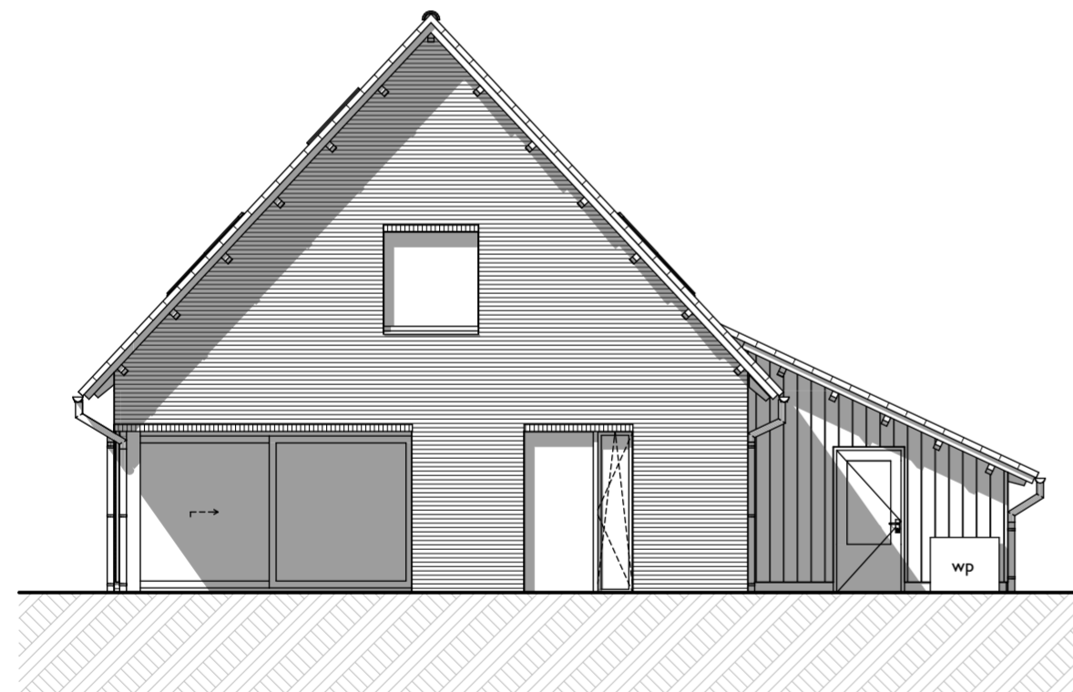
bnr 1/2 Achtergevel
