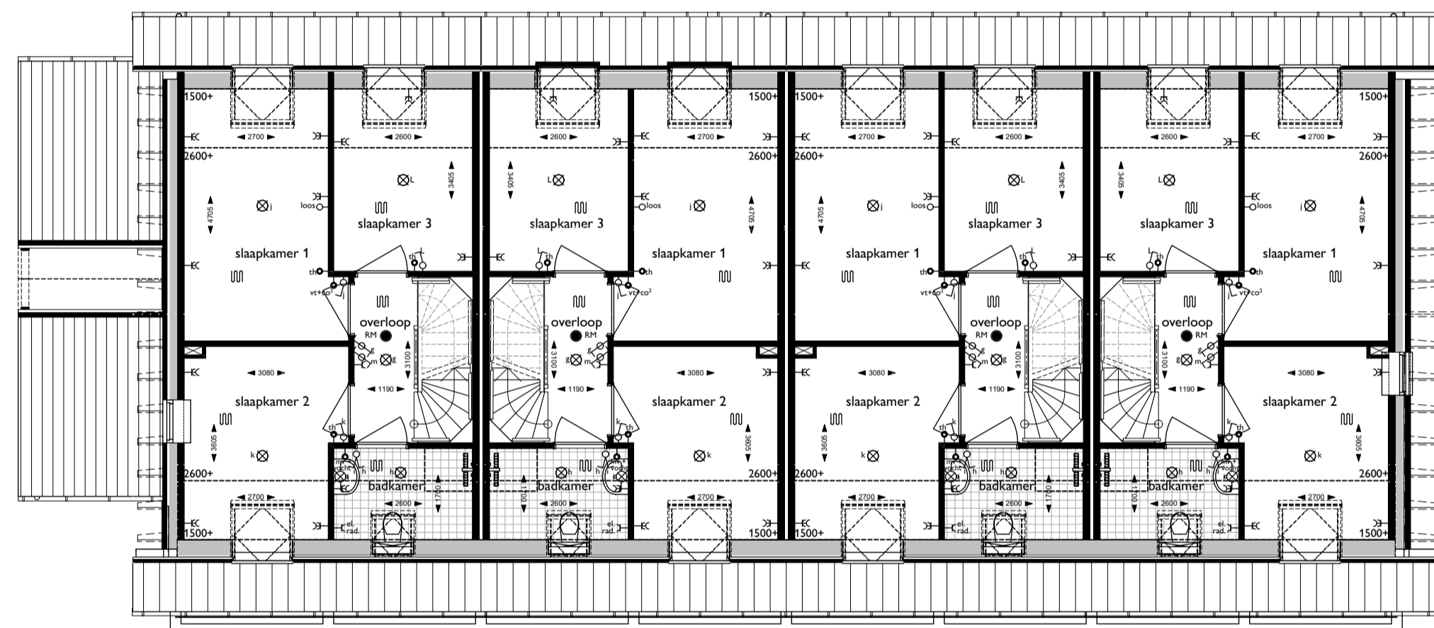
Eerste verdieping
