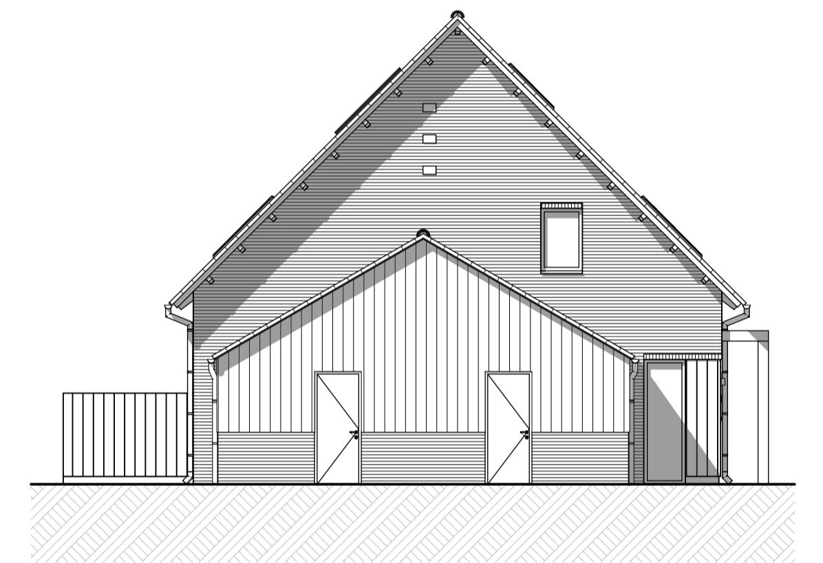
Linkergevel
