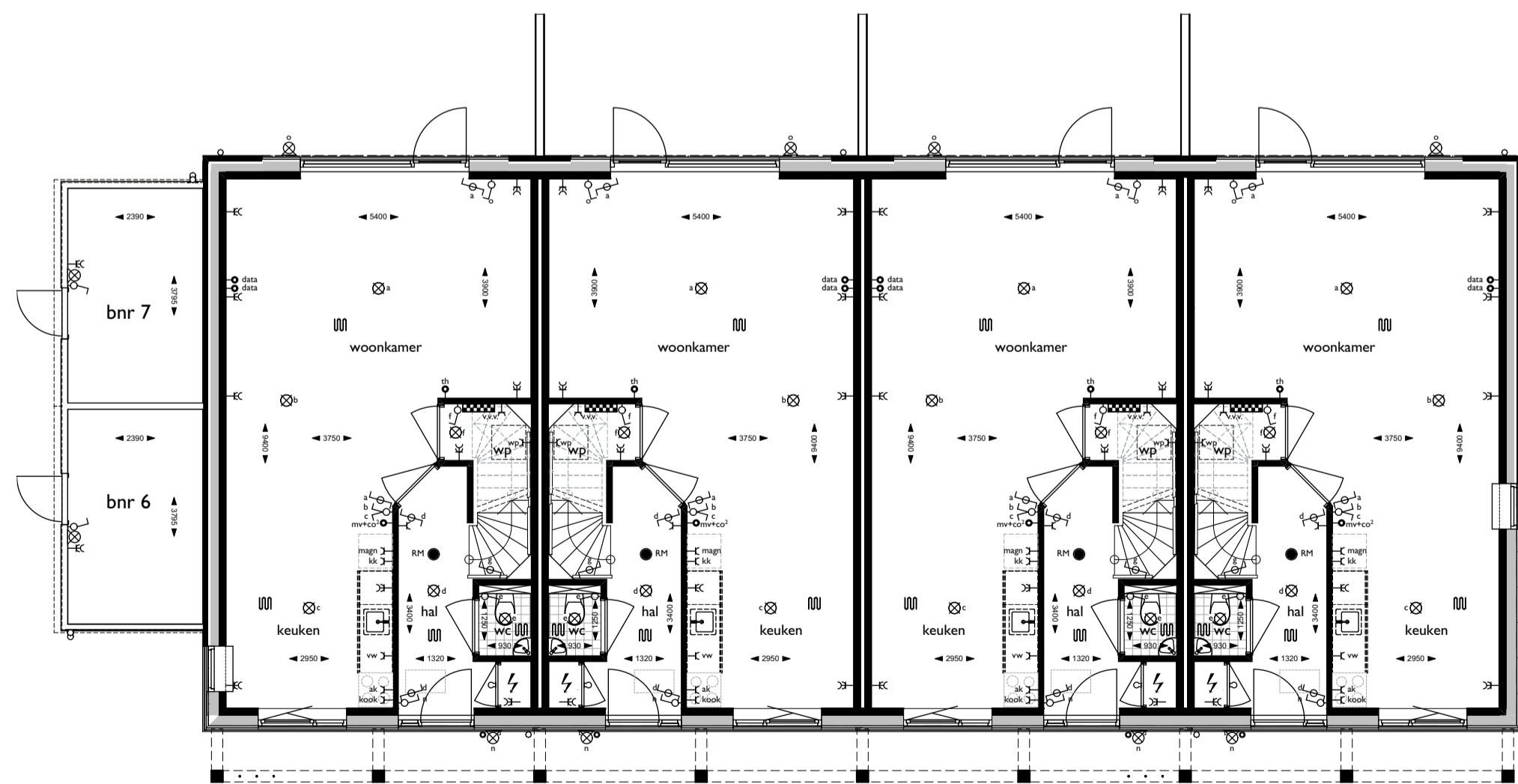
Begane grond
