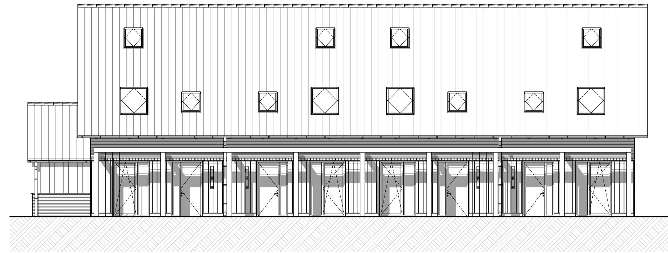
Voorgevel
