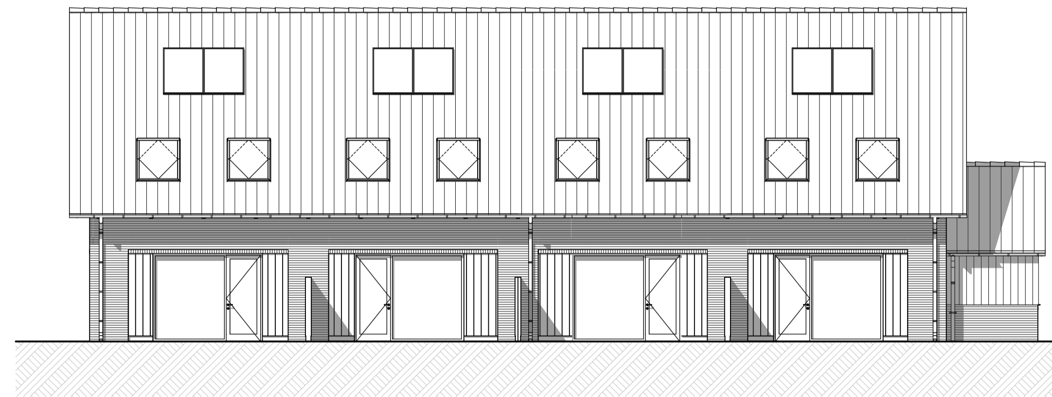
Achtergevel
