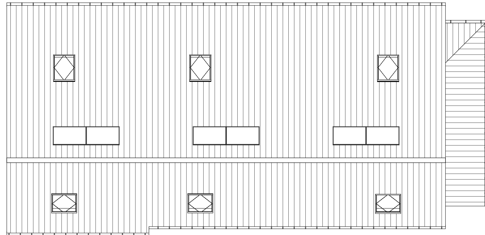
Dakaanzicht
