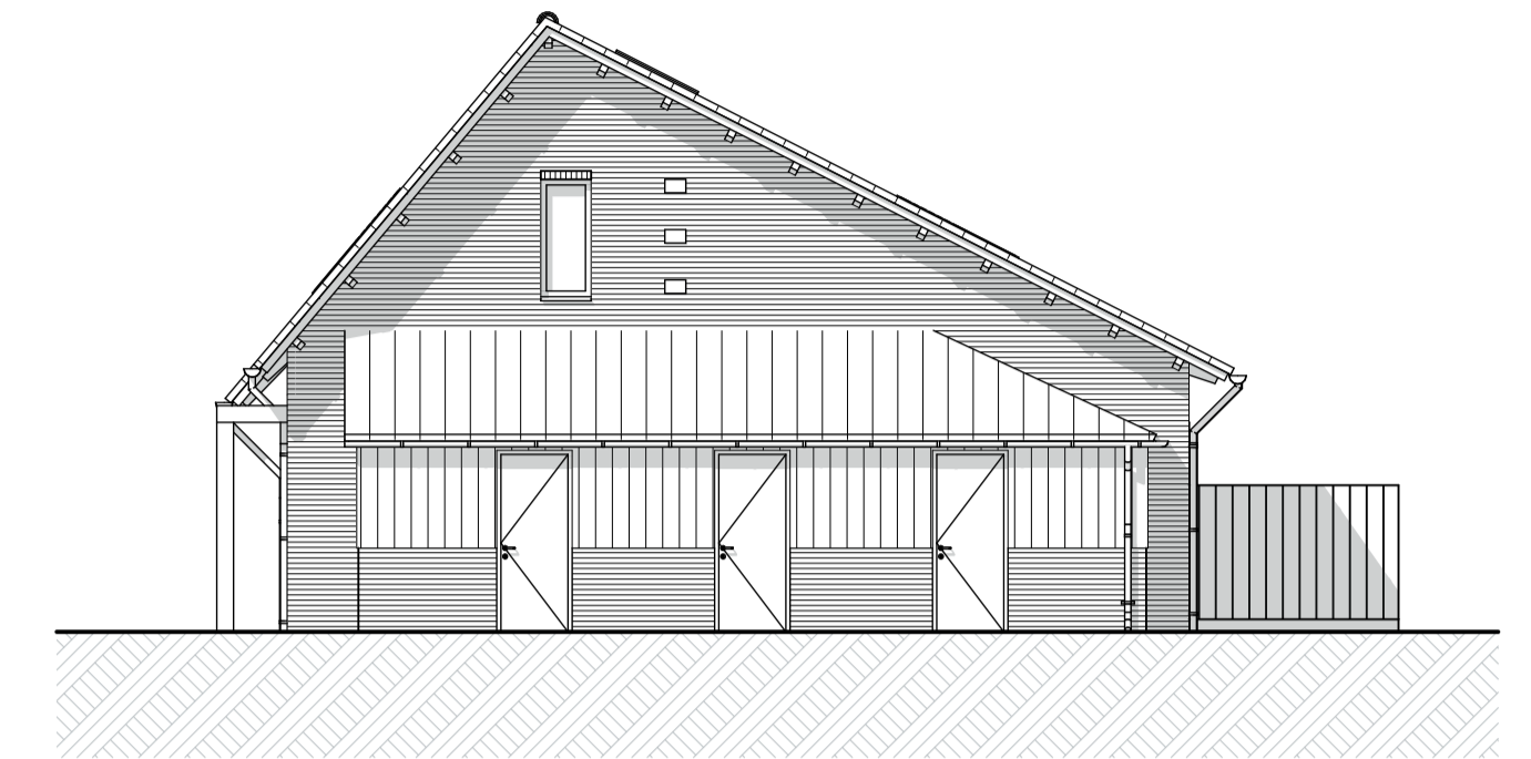
Rechtergevel
