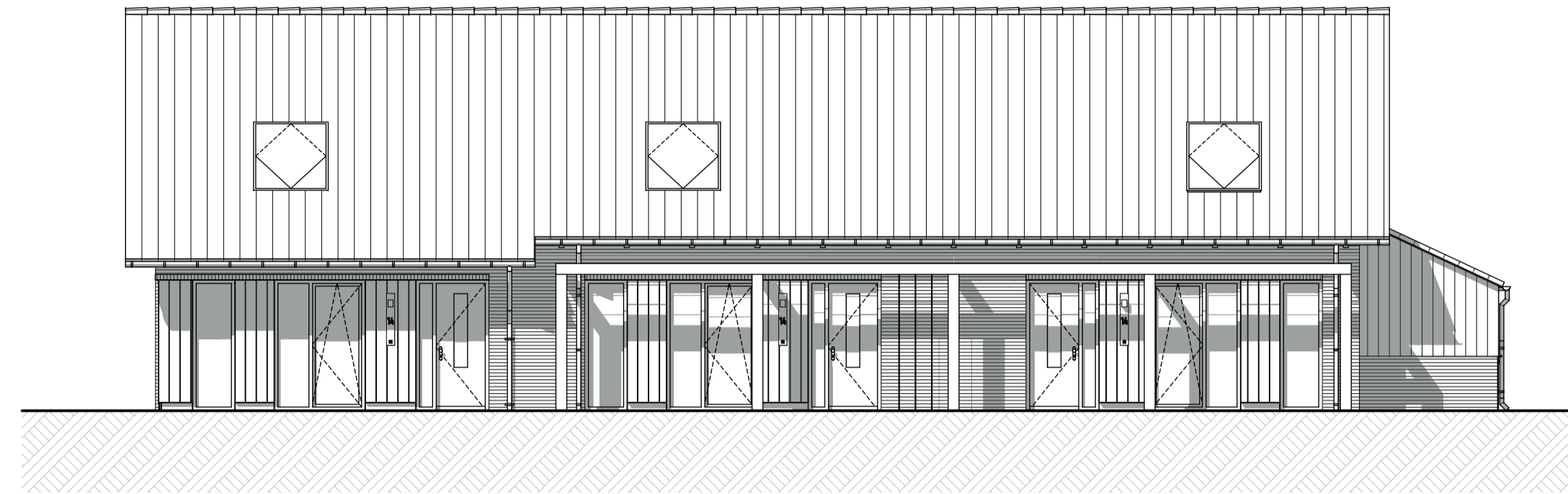
Voorgevel
