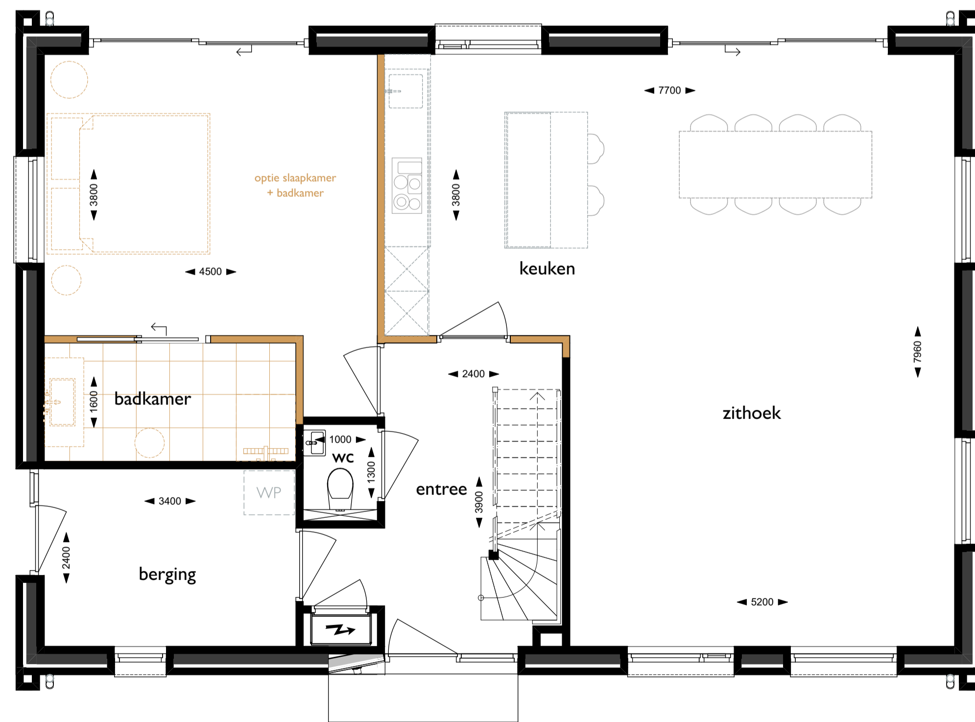
Begane grond
