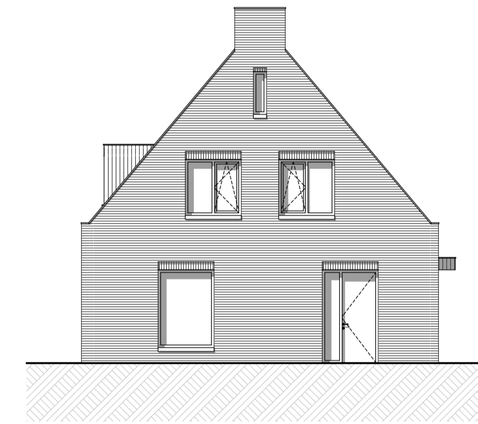
Linkergevel
