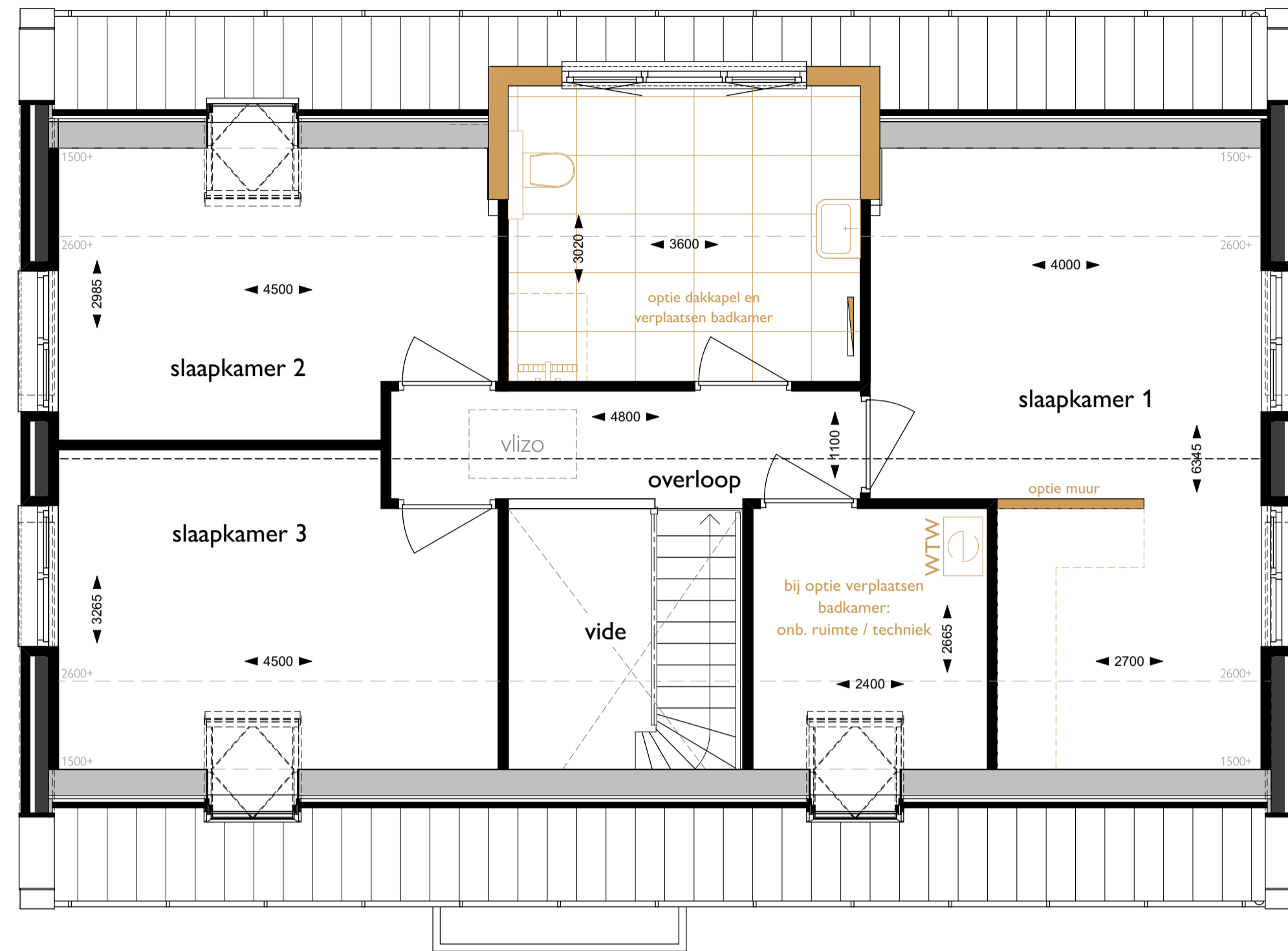
Verdieping
