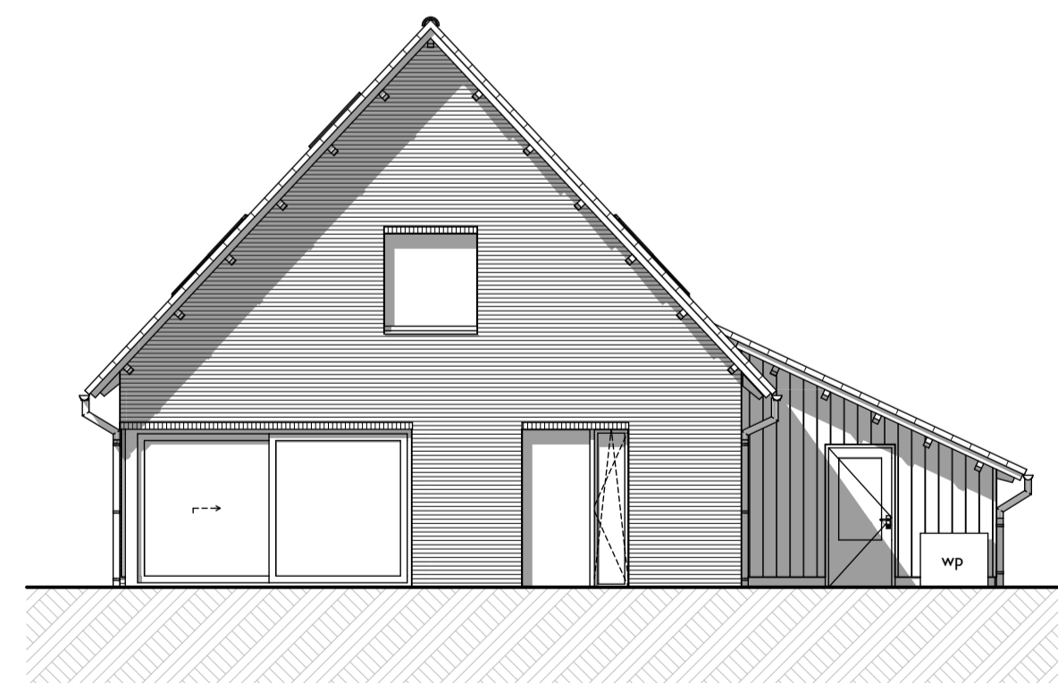
Achtergevel - optie terras dichtbouwen
