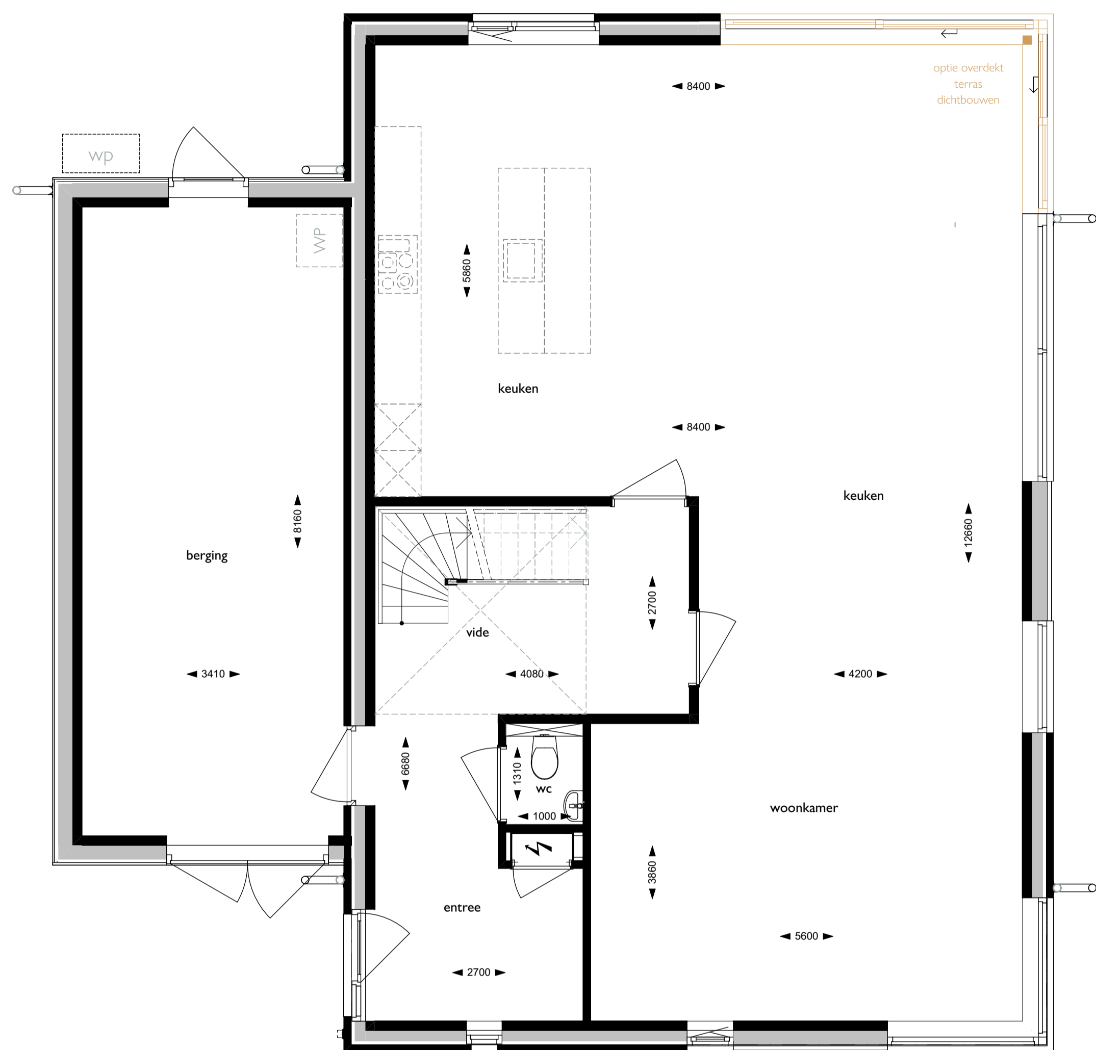
Begane grond - optie terras dichtbouwen
