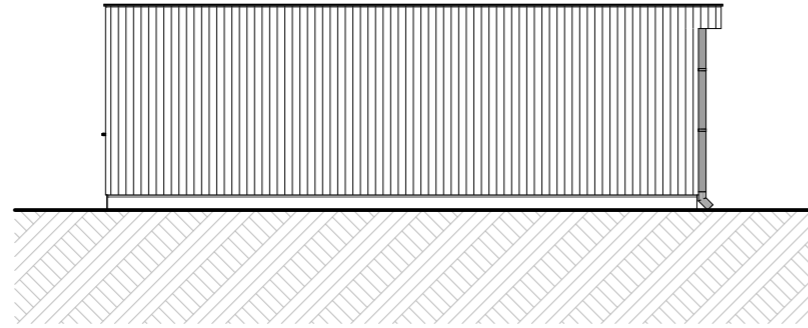
Rechtergevel carport
