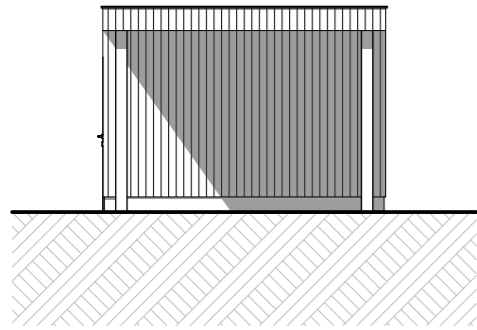
Voorgevel carport
