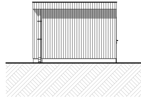
Achtergevel carport
